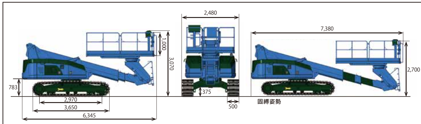
外觀圖
