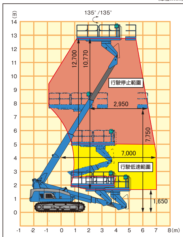
工作範圍圖
